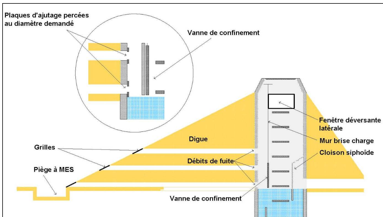
Figure 16 : Ouvrage de régulation et de traitement en sortie de bassin tampon (cas d'un lotissement)
