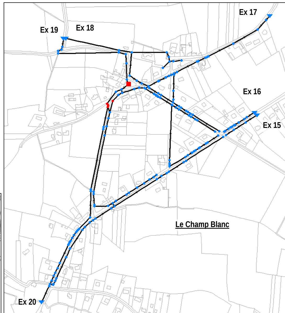
Figure 21 : Localisation des débordements résiduels pour une pluie trentennale en situation projet – Secteur des hameaux
