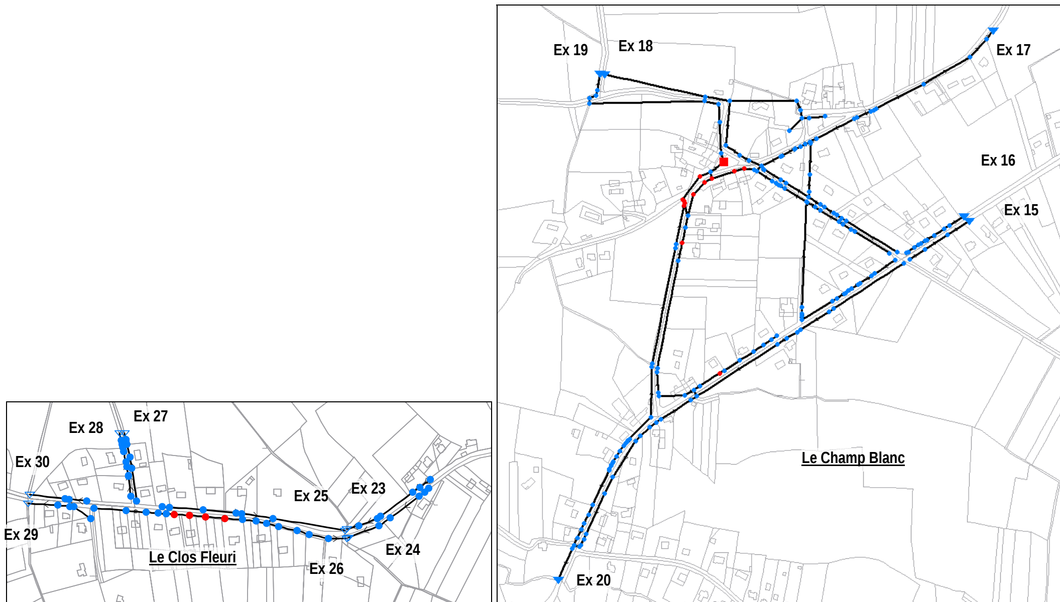
Figure 22 : Localisation des débordements résiduels pour une pluie centennale en situation projet – Secteur des hameaux
