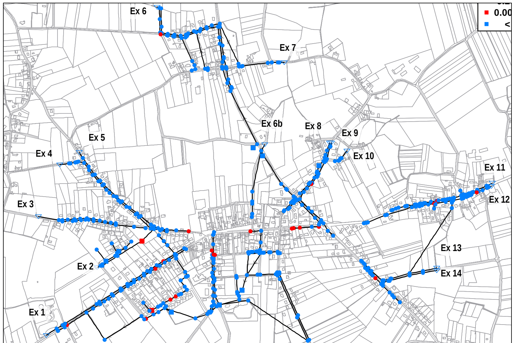
Figure 19 : Localisation des points de débordement résiduels pour une pluie trentennale en situation projet – Secteur du bourg
