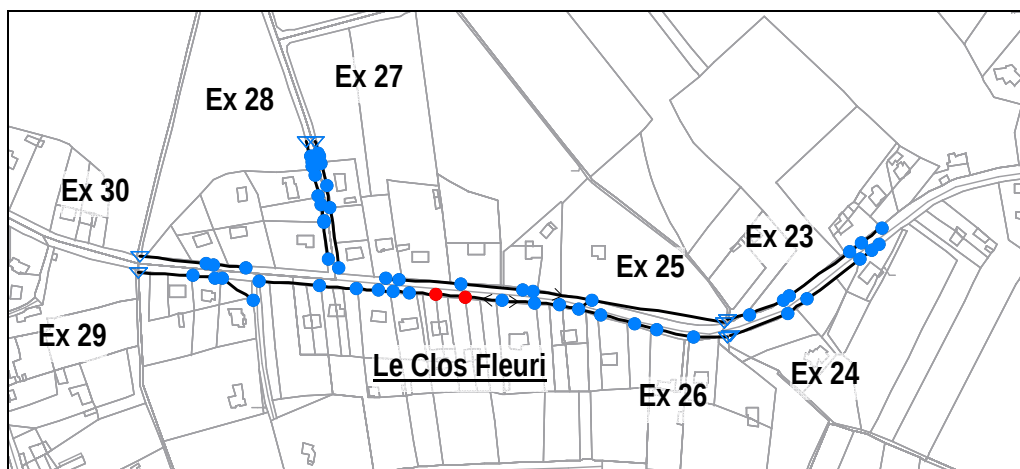
Figure 21 : Localisation des débordements résiduels pour une pluie trentennale en situation projet – Secteur des hameaux
