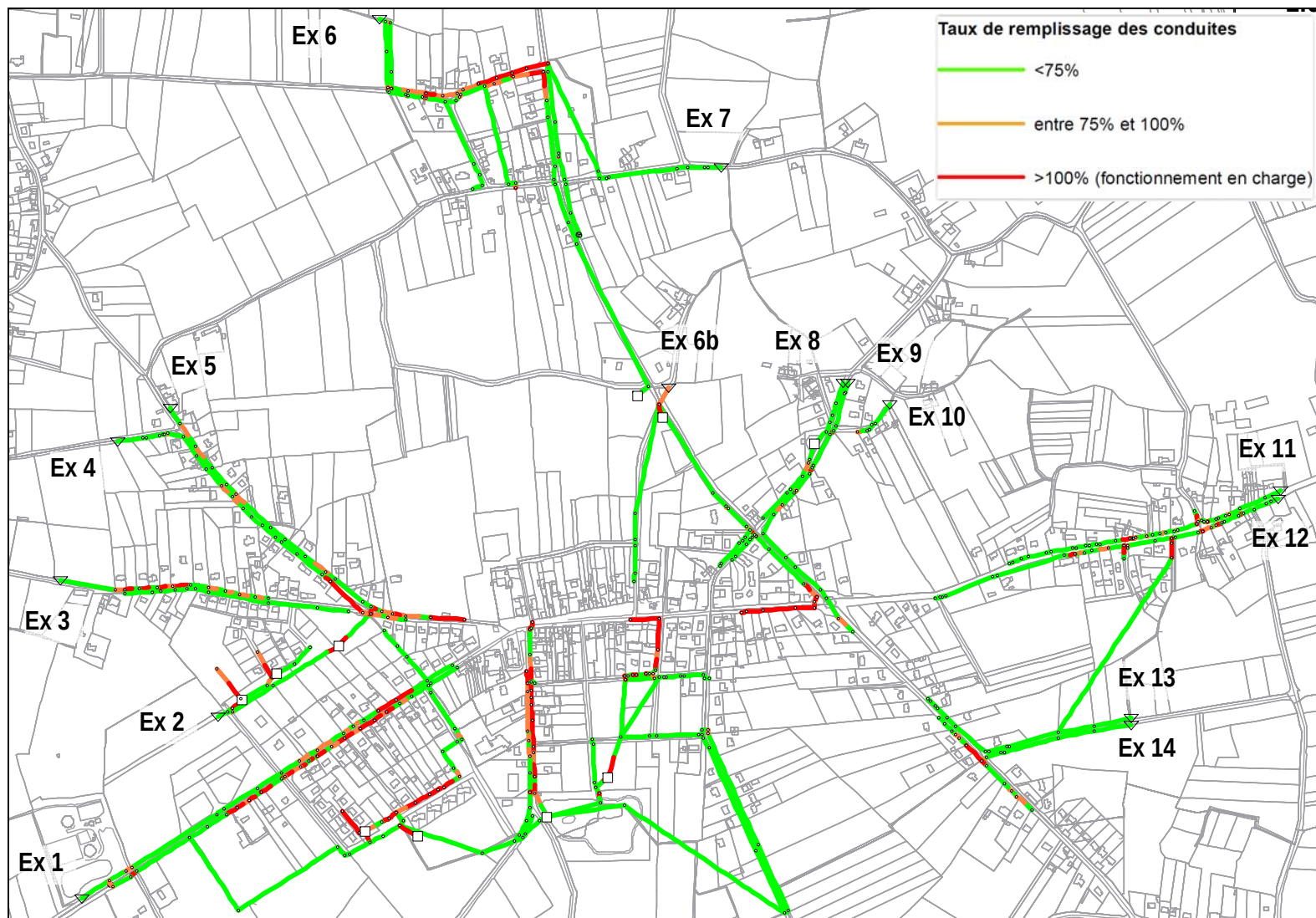
Figure 17 : Taux de remplissage des conduites et absence de débordements pour une pluie décennale en situation projet – Secteur du bourg
