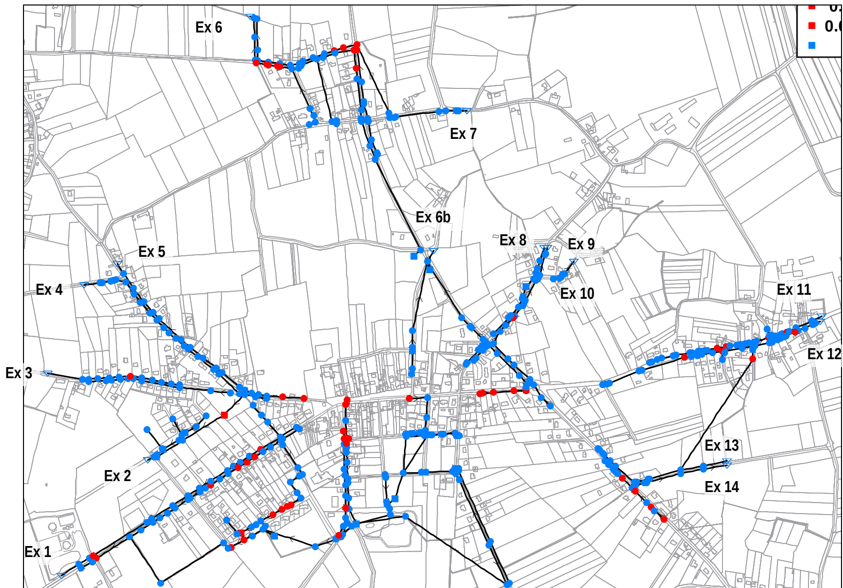
Figure 20 : Localisation des points de débordement résiduels pour une pluie centennale en situation projet – Secteur du bourg
